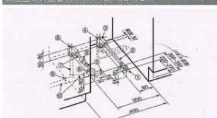
床立上げの配管例(キッチン奥行850mmの場合)
