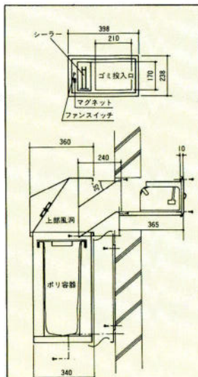
写真は右仕様 BD-500・R/L(壁面投入ロタイプ) 445(W)×340(D)×918(H) ¥68,000(工事費別)
