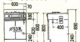
ガスキャビネット 60GC
