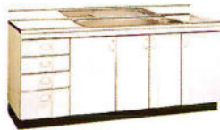
流し台(ジャンボ水槽) CW-180J 1800×560×800 ¥119,500 左・右水槽がございます。
