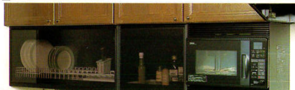
食器乾燥庫 BUC-SD90A ¥79,000 900×320×400 AC100V・消費電力 300W 温風通風式 ・食器収納約6人分
