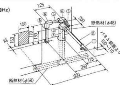
①床立上げの配管例(排水管を上にしてください)
