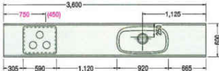
3600(ジャンボシンク)R
