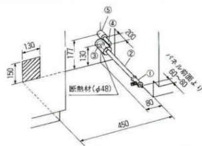
②壁出しの配管例(配水管を上にしてください)
