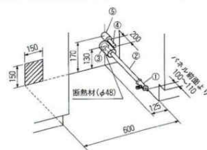
②壁出しの配管例(排水管を上にしてください)
