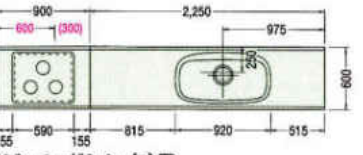
3600(ジャンボシンク)R
