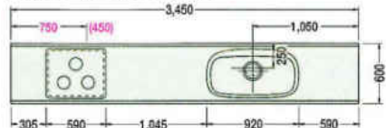
3450(ジャンボシンク)R
