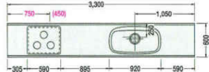
3300(ジャンボシンク)R
