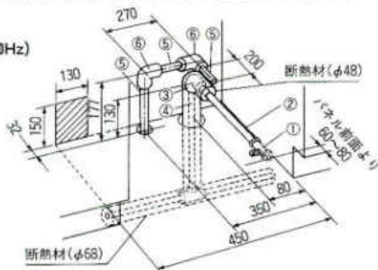
①床立上げの配管例(配水管を上にしてください)
