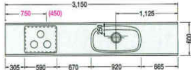
3150(ジャンボシンク)R
