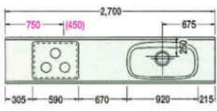
2700(ジャンボシンク)R
