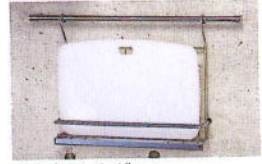
まな板ホルダー TU-4001 ¥13,000 開口420mm×奥行110mm×高さ350mm
