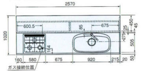
PC-255J
