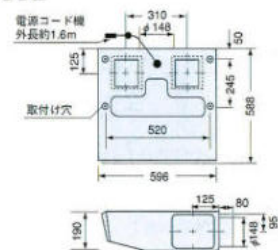
FH-602
