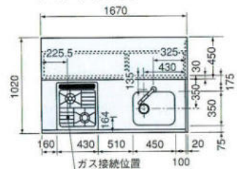
PC-165S
