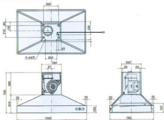
HDR-1251S
