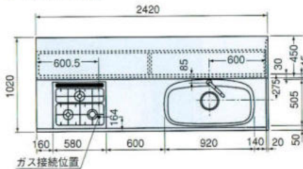
PC-240J
