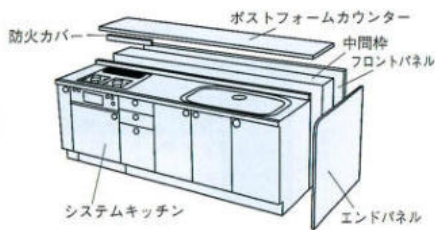
PC-240J
