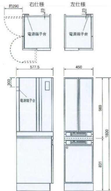
N-451MVD (ミドル)
