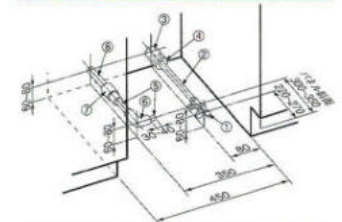
壁出しの配管例 (キッチン奥行65cmの場合)
