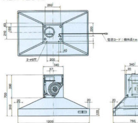
HDR-1251S
