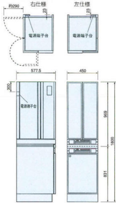
N-451MVD (ミドル)
