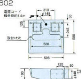
FH-602
