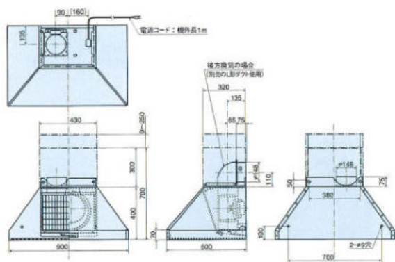
TPR-3S-903S
