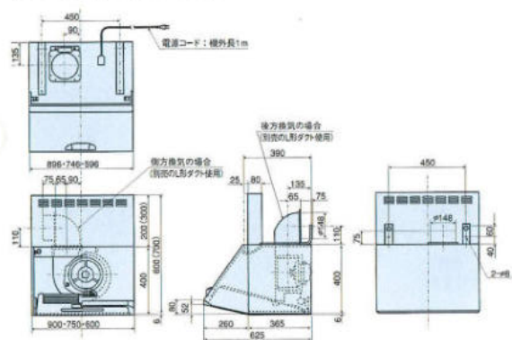
FCR-3R-903/753/603 (9037/7537/6037)
