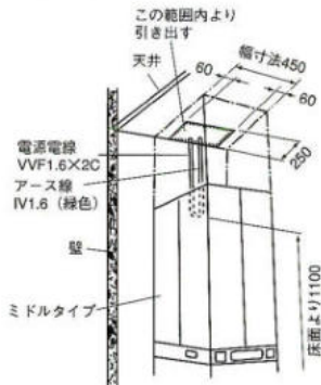
N-451MVD (ミドル)
