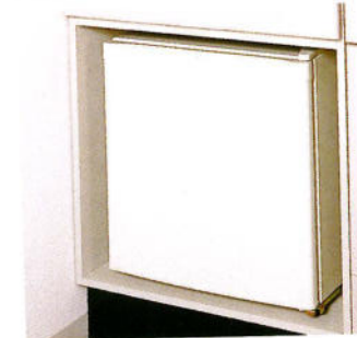
冷蔵庫 幅460×奥行496×高さ488mm ¥39,500 有効内容量 40L ※冷蔵庫の扉は右開きのみです。
