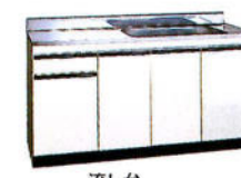
流し台 SW-150S 1500×550×800 ¥56,000 左・右水槽がございます。
