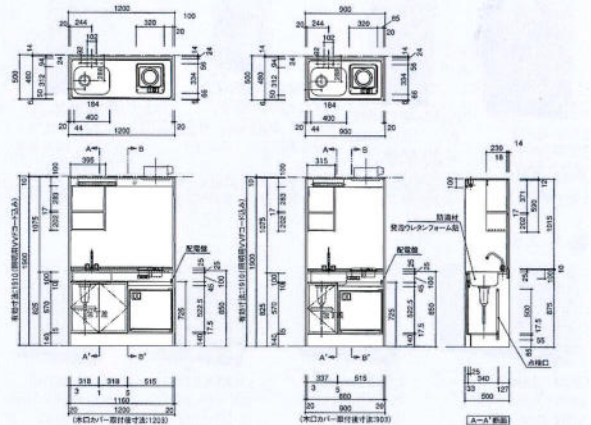
MKT-120A1JL MKT-90A1JL
