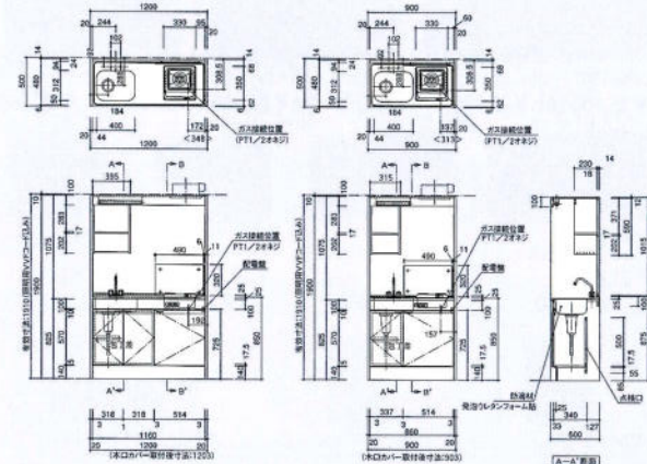
MKT-120BGL MKT-90BGL
