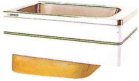
和洋折衷埋込式2方半エプロン(右・左有) HEP-1202 ¥121,000 SEP-1202(立上り付) ¥123,200 間口11200×奥行730×高さ625% (満水量285ℓ) ※立上りの高さ寸法は20%です。
